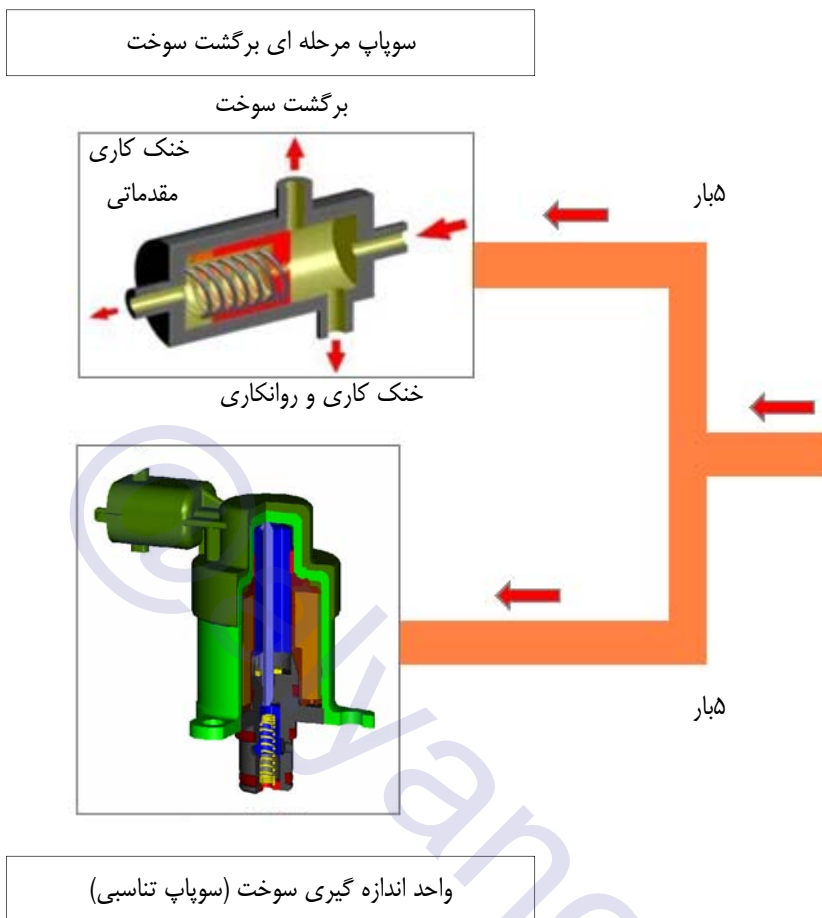
شکل ۶-۱: مسیر سوخت هبار
